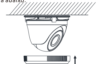
Figura 2-10 Fixação do anel de recorte na câmera
